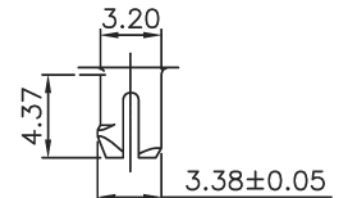
DETAIL Y
